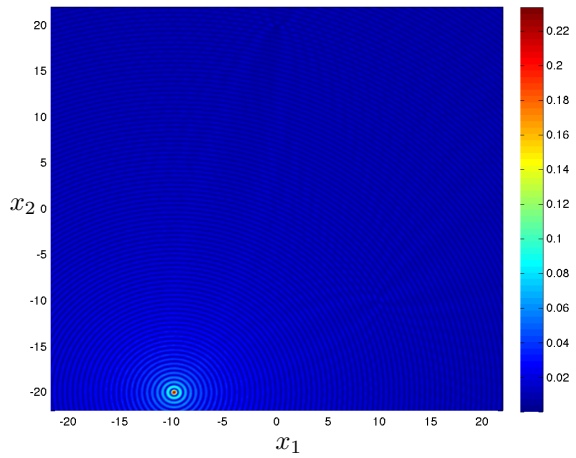
(d) Amplitude of the third Herglotz wavefunction
