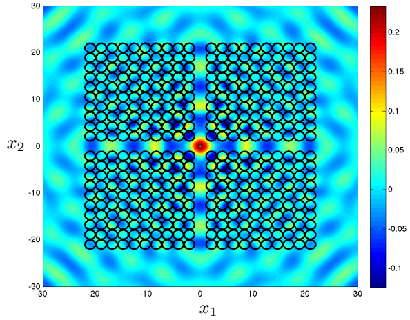
(d) Penetrable problem: \Im(u^{\text{tot}})
