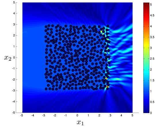
(d) Sound-soft problem: |u|
